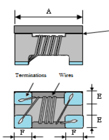
外观尺寸
